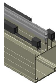
Montant 92mm Moment d'inertie : 83 cm 4
